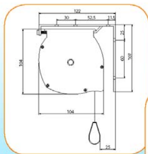
Disegni Tecnici del cassetto Ellipse
